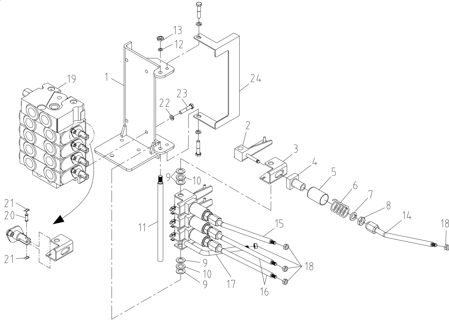
벨브 스텐드 세트 Fig. 3-3-1 SCS744L VALVE STAND SET
