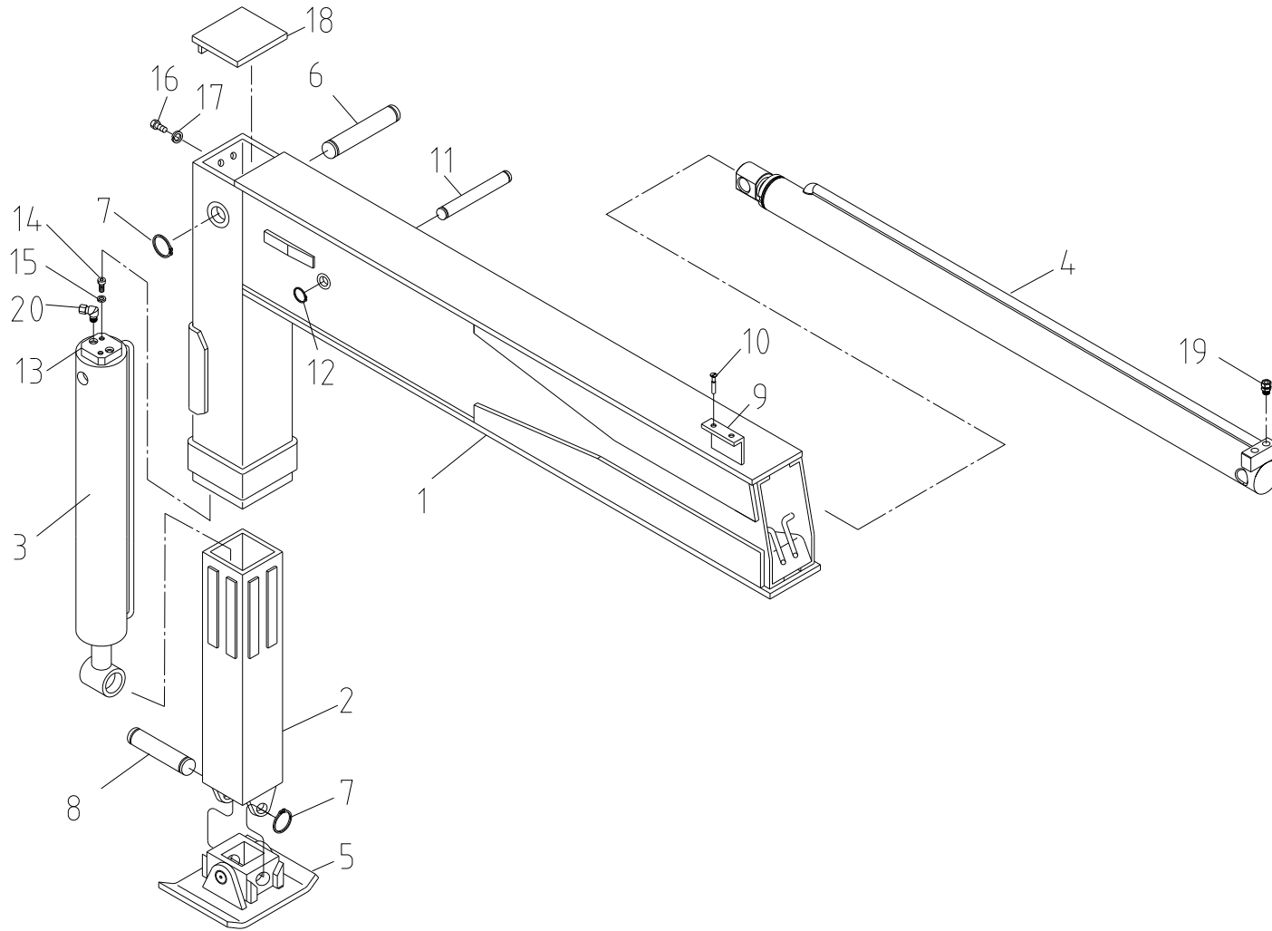
아우트리거 조립체 Fig. 4 SCS744L OUTRIGGER ASS'Y
