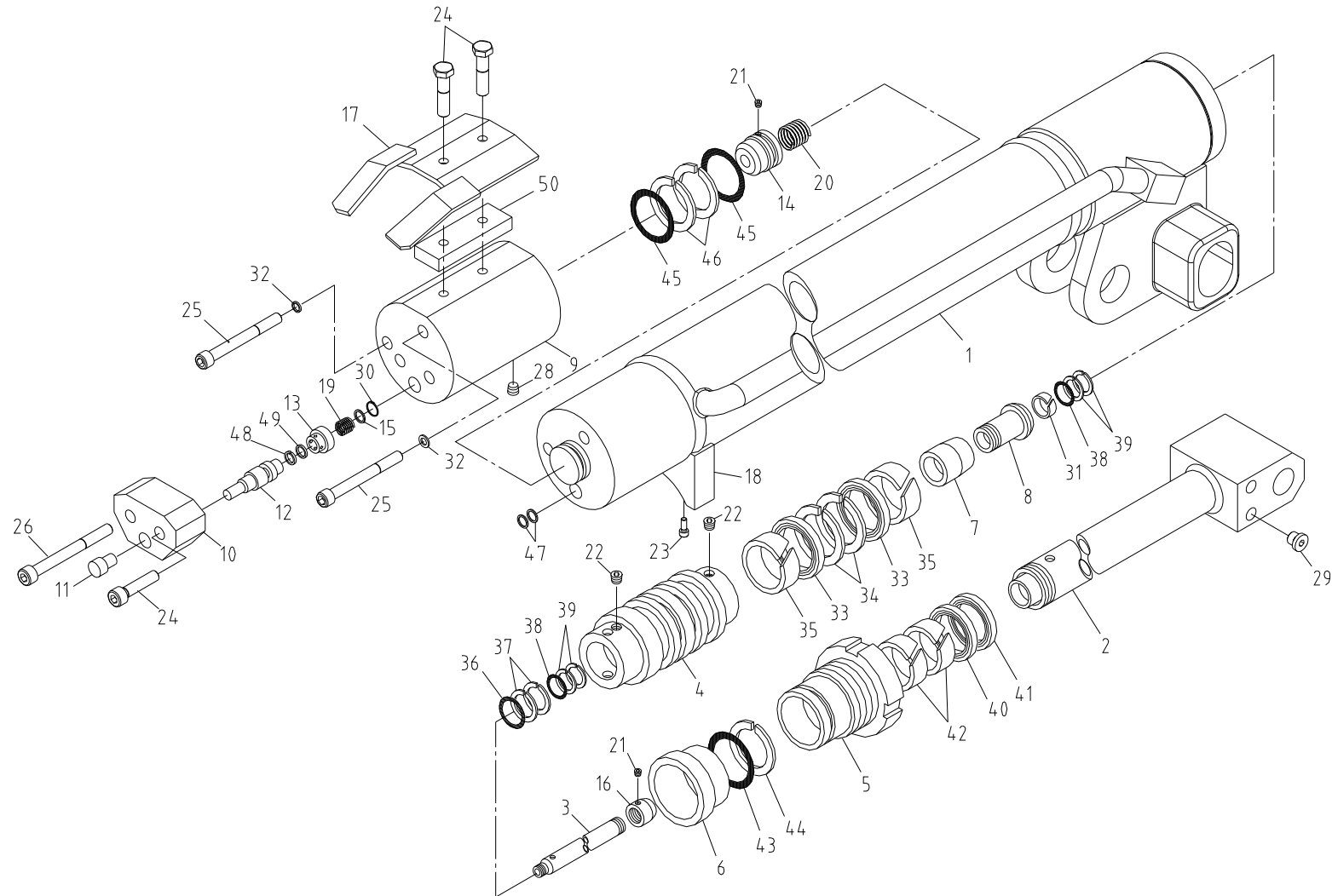
텔레스코픽 실린더(1 단) 조립체 Fig. 1-1-1 SCS744L TELESCOPIC CYL'(1st) ASS'Y
