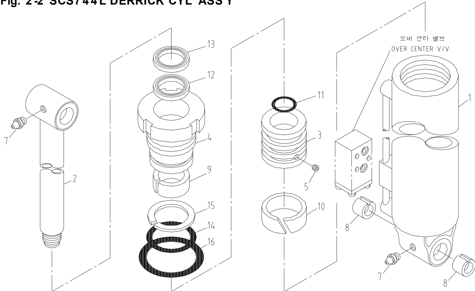
데릭 실린더 조립체 Fig. 2-2 SCS744L DERRICK CYL' ASS'Y
